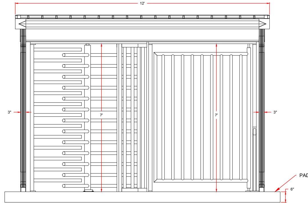
ELEVATION (entrance side typ.)
