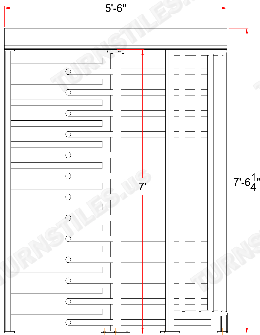
ELEVATION
