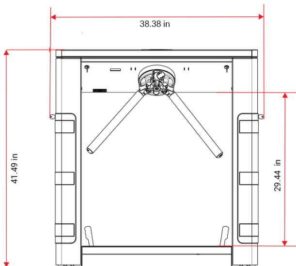
CatRax Portable
