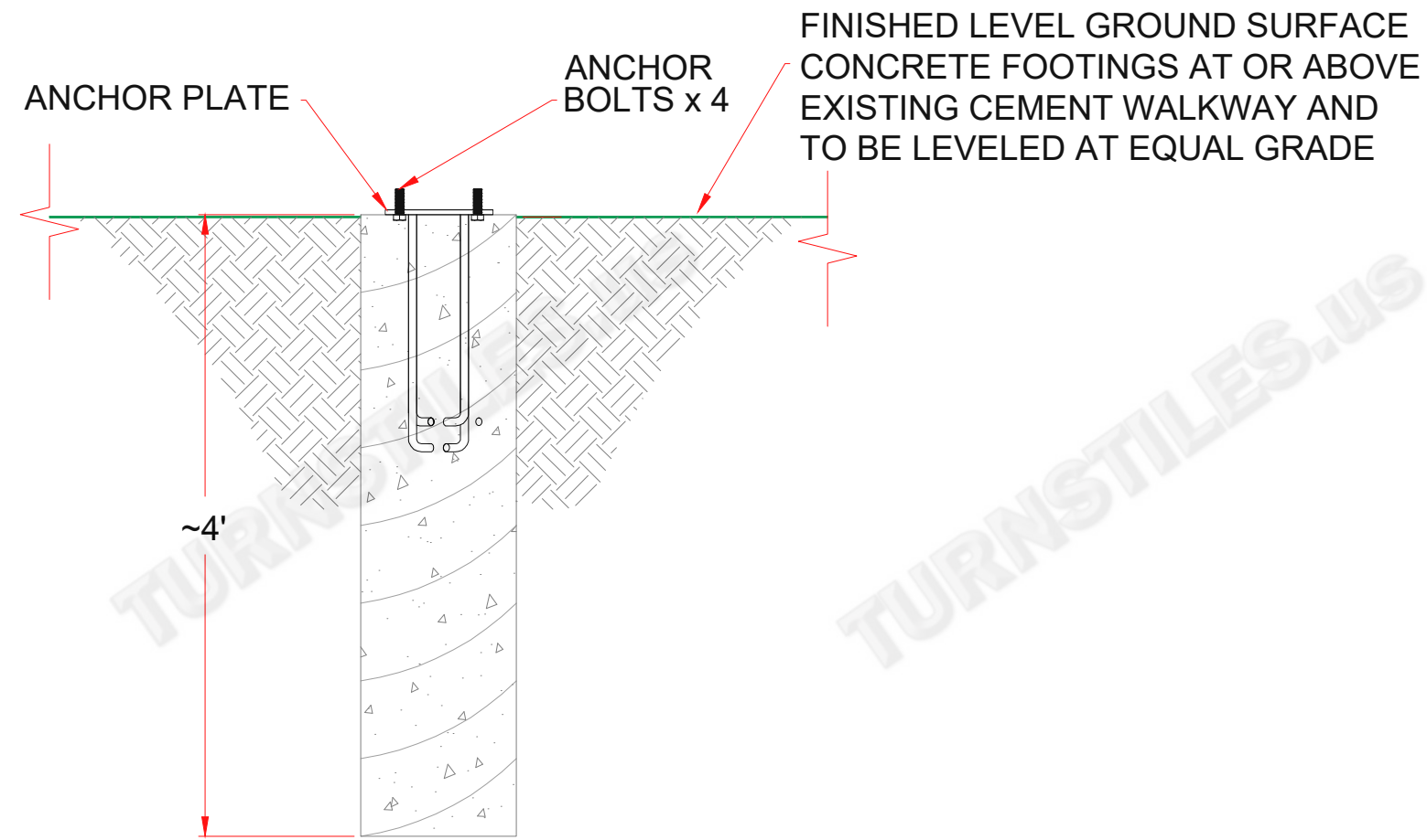
ELEVATION
