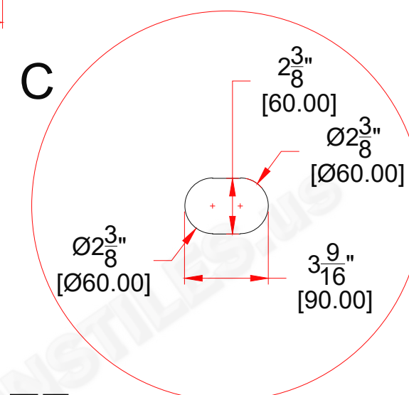
TEMPLATE DIMENSIONS
