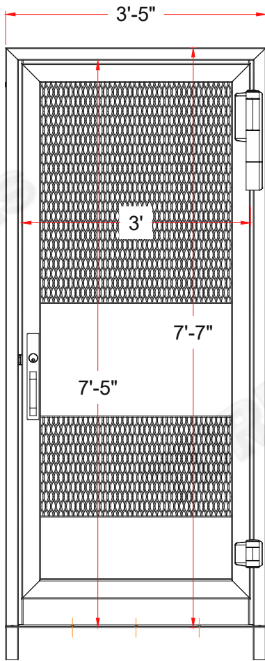
ELEVATION
