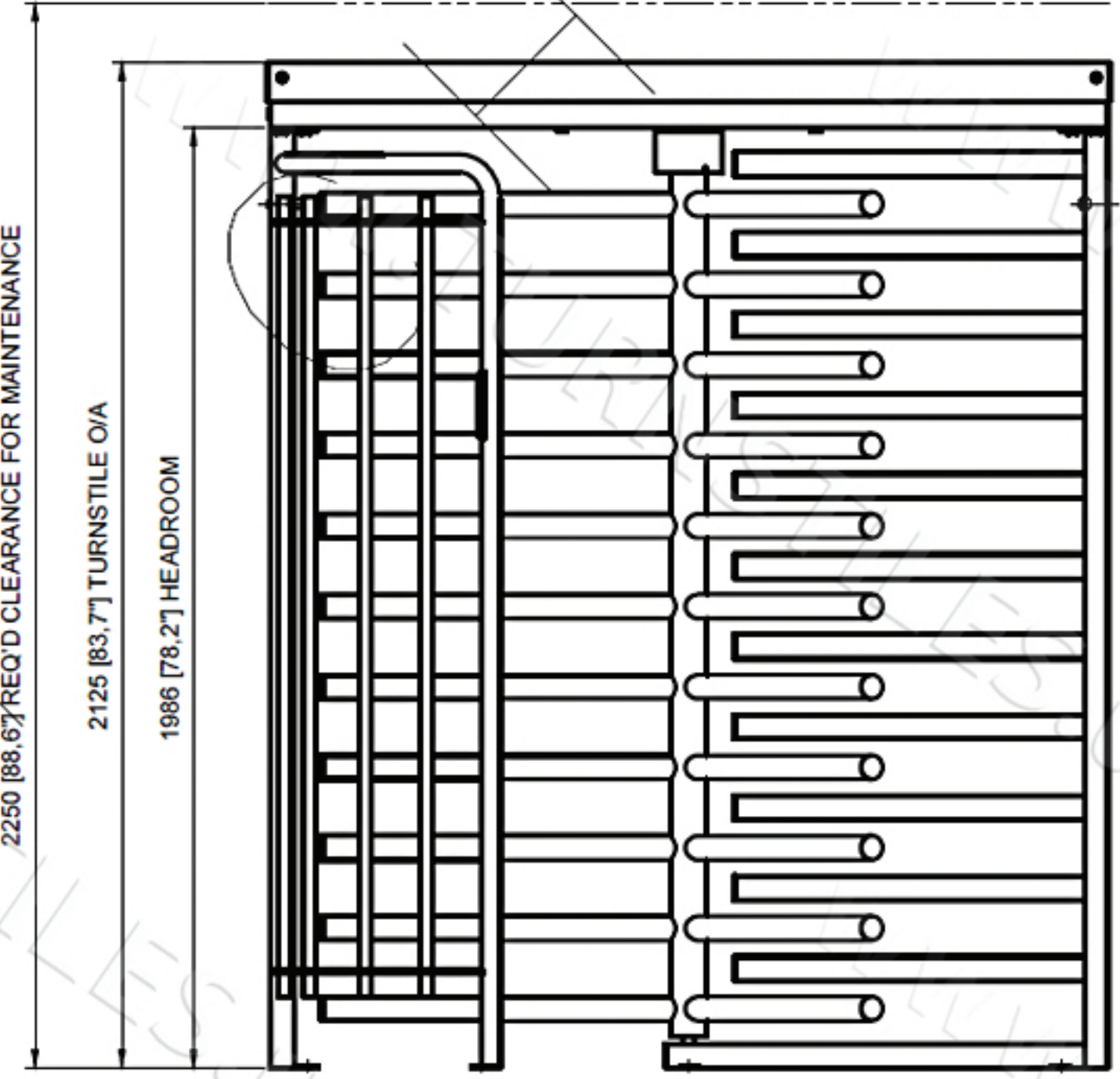
ELEVATION
