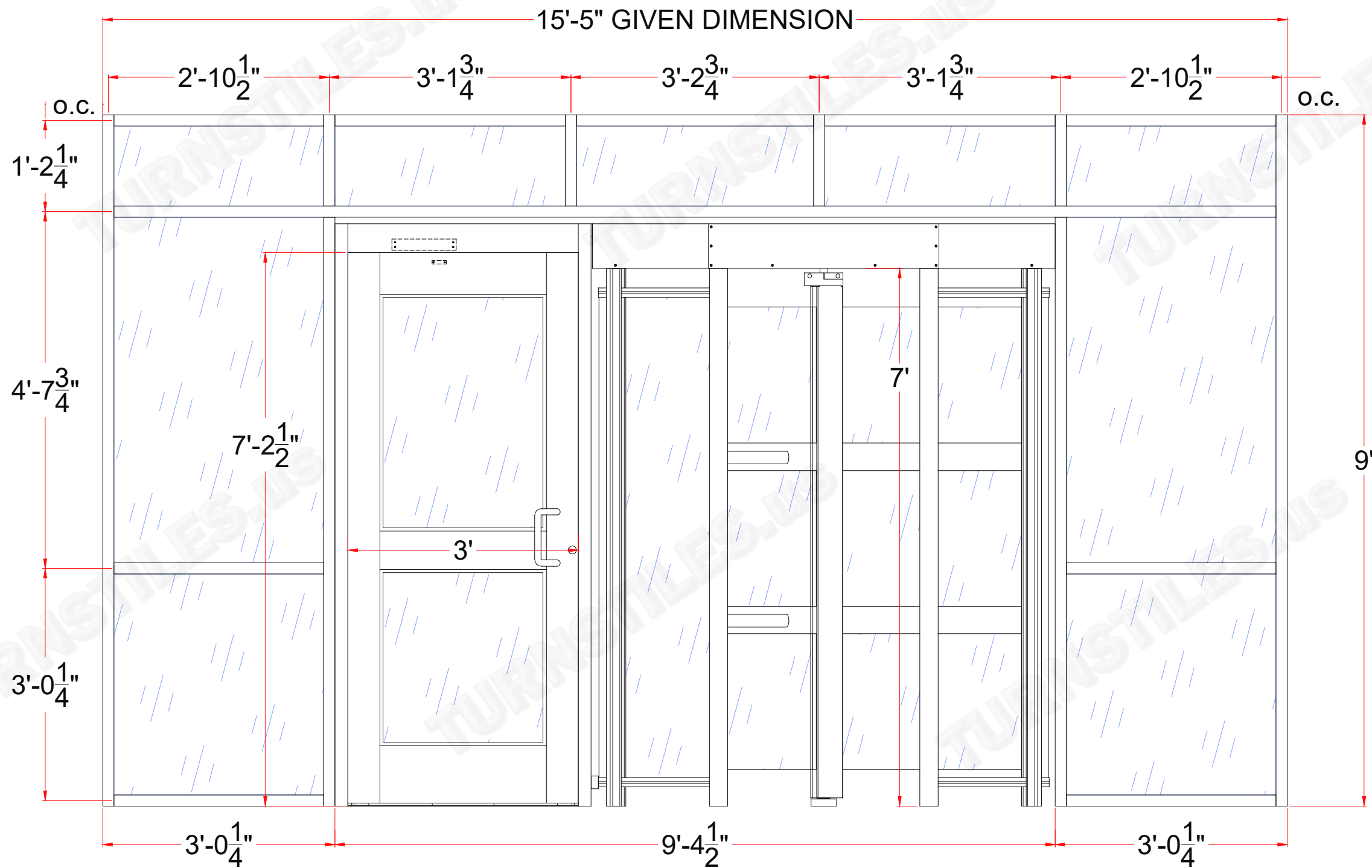
ELEVATION NON - SECURE SIDE
